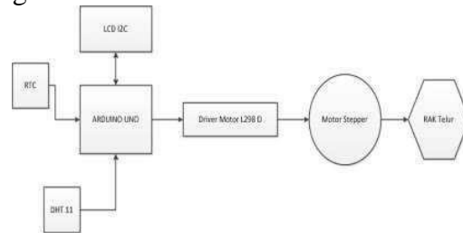
Gambar 2 Diagram Blok Sistem Pemutaran Rak Telur
